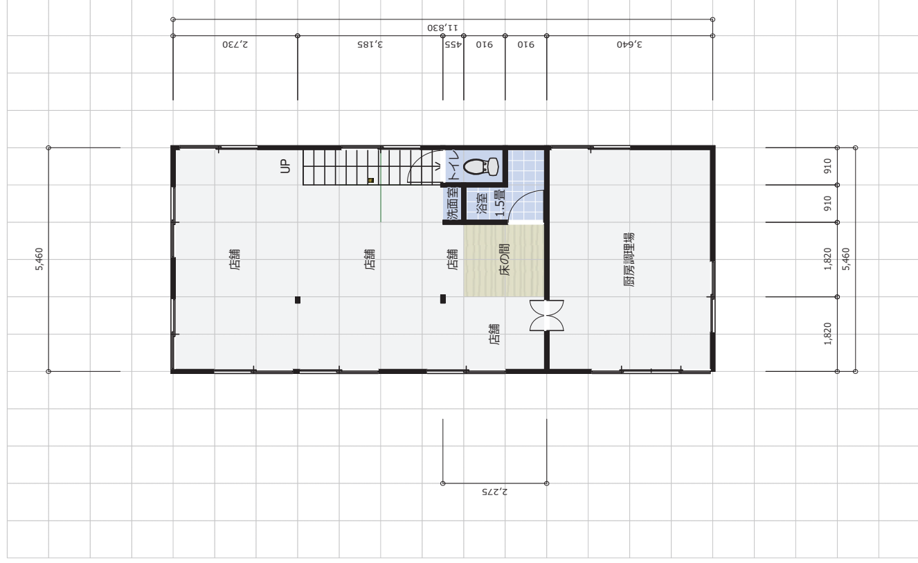
1階縮尺 1/150
