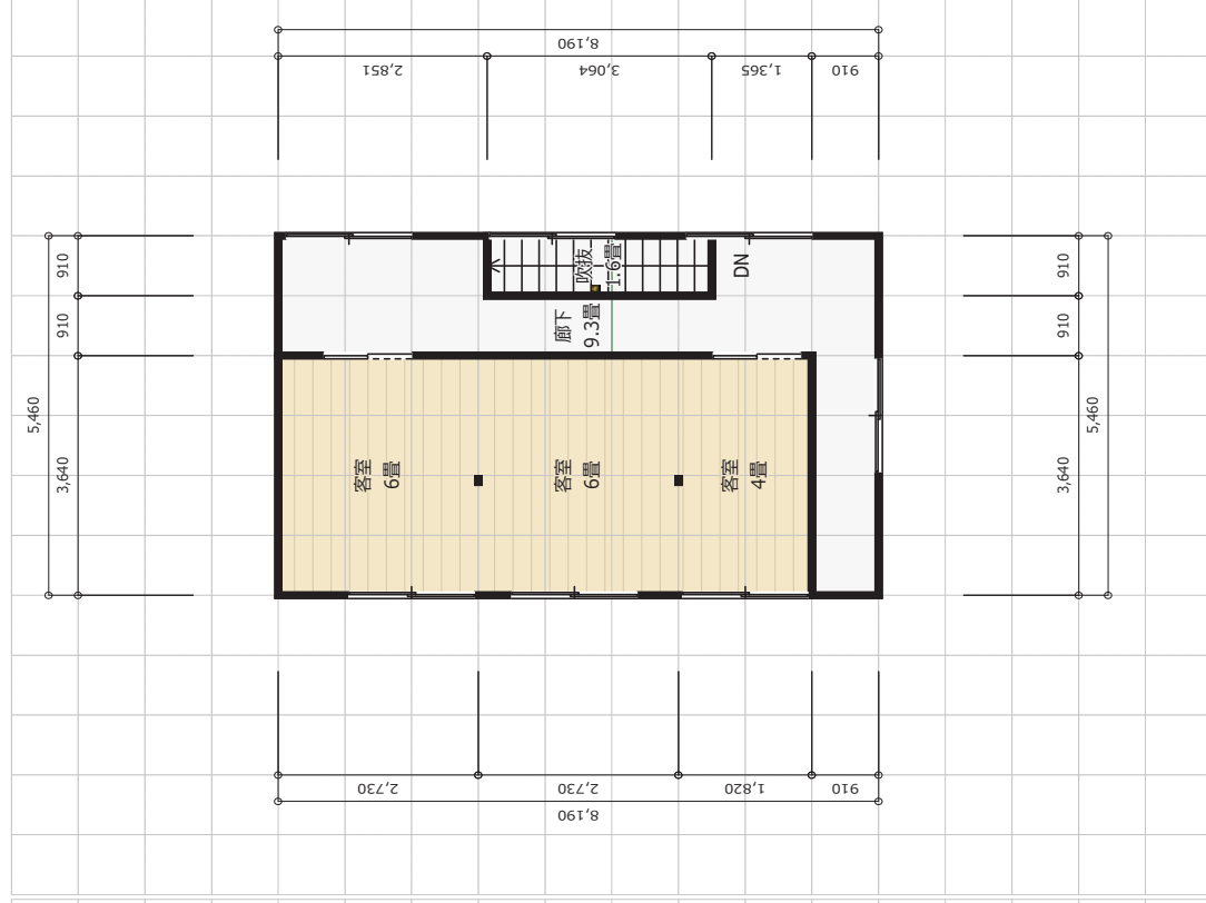
2階縮尺 1/150
